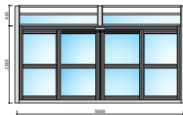
Automatische Schiebetür
