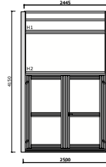
Doppelflügel Nottür
