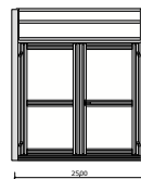
Doppelflügel Nottür
