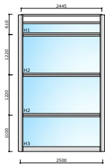
Glasfüllung
